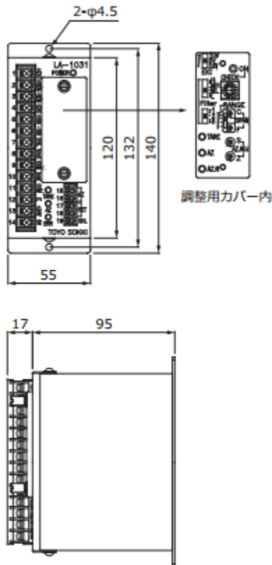
外形寸法 Outline Dimensions (mm)
